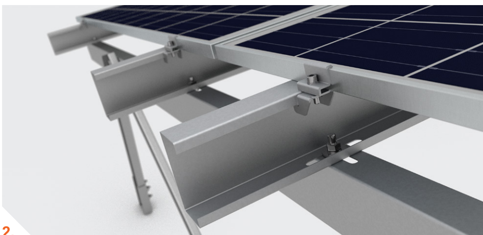
2. Uchytení panelů na podélné profily
